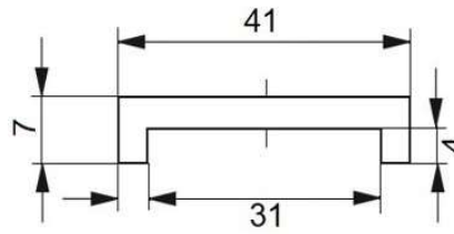
PERFIL "Z" 20X8
