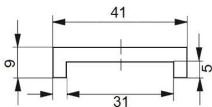
PERFIL apoyo tipo "U4" 45x9
